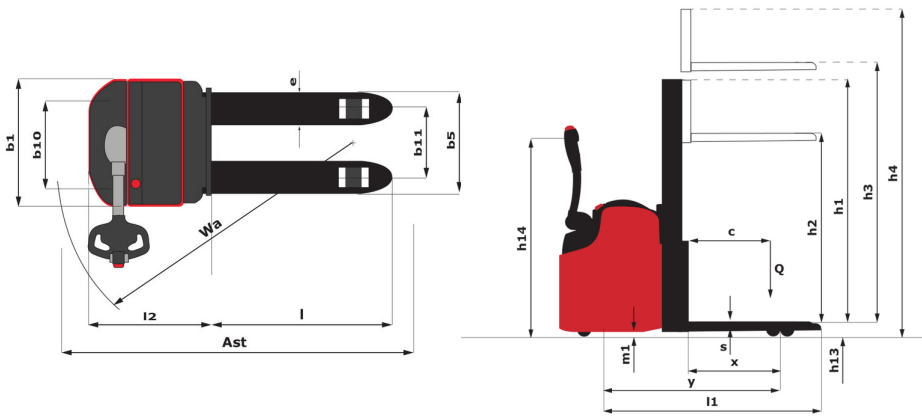
ES 725 - габаритный чертеж
