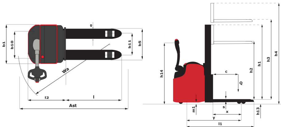
ES 725 - Tekening met afmetingen
