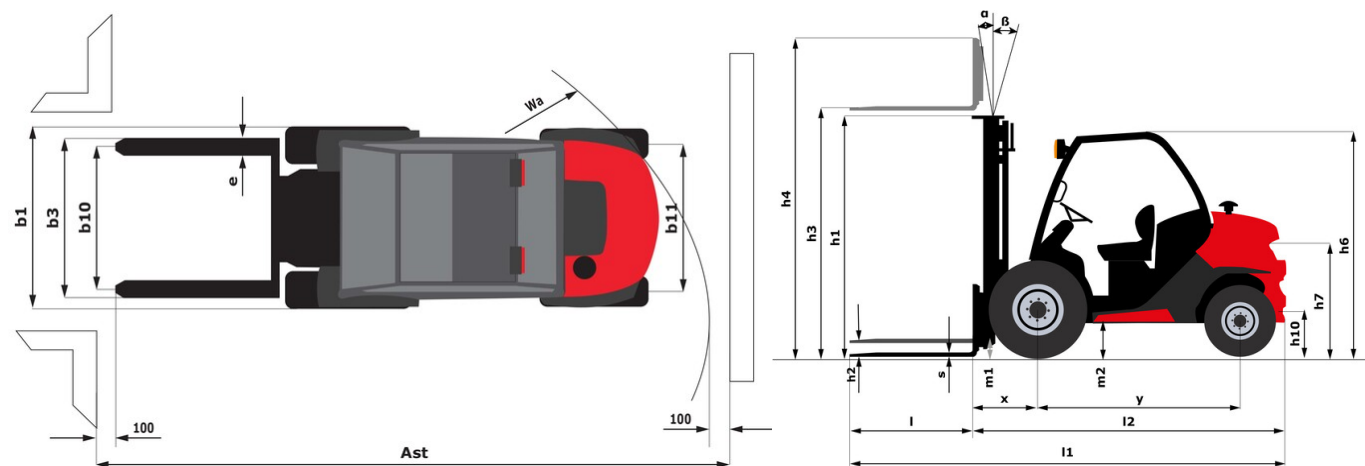
MC-X 30-2 - Schémas d'encombrement
