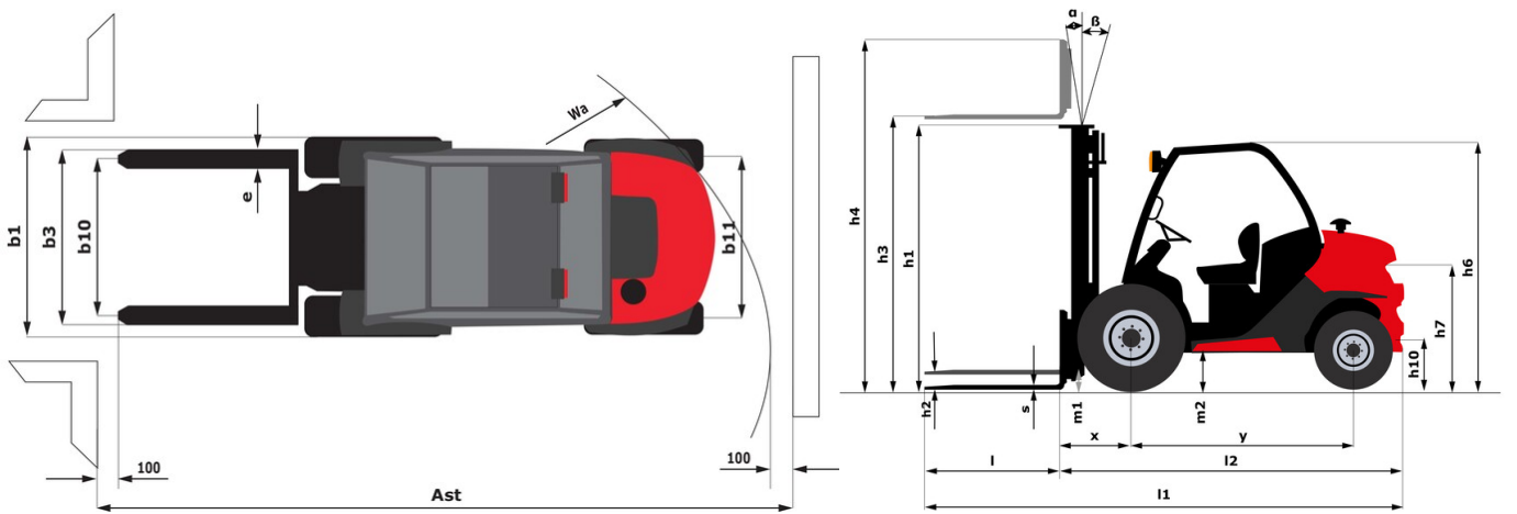
МС-Х 30-2 - габаритный чертеж
