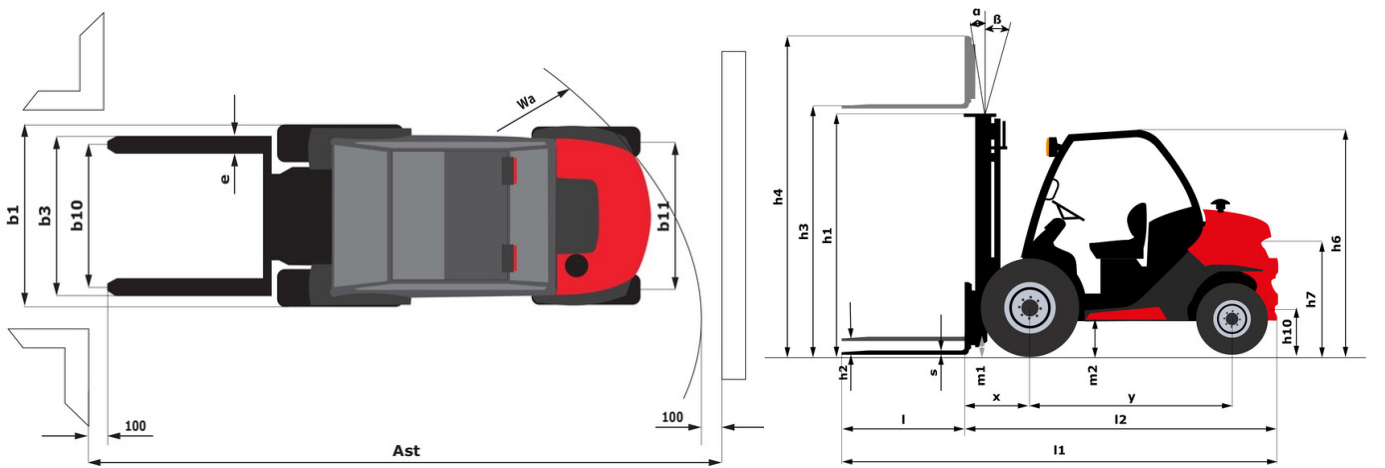
МС-Х 30-4 - габаритный чертеж
