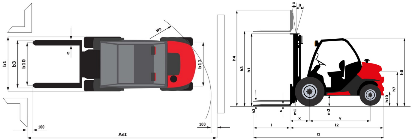
MC 30-4 ST5 - Tekening met afmetingen
