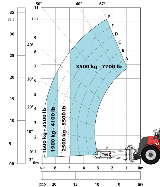
Машина на колесах с захватом для шин ТН 51, метрическая система мер
