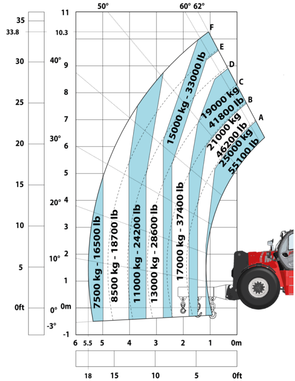
Machine op banden met 3-hook giek 25000 kg (Metrisch)
