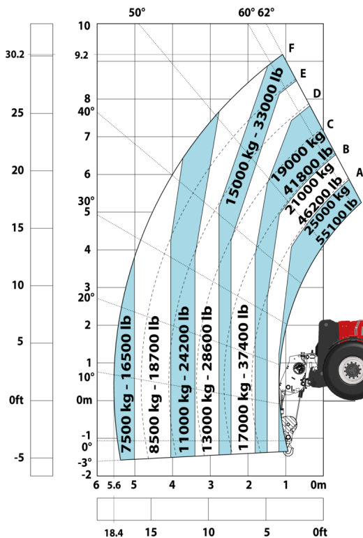
Maszyna na oponach z wciągarką 25000 kg (metryczne)
