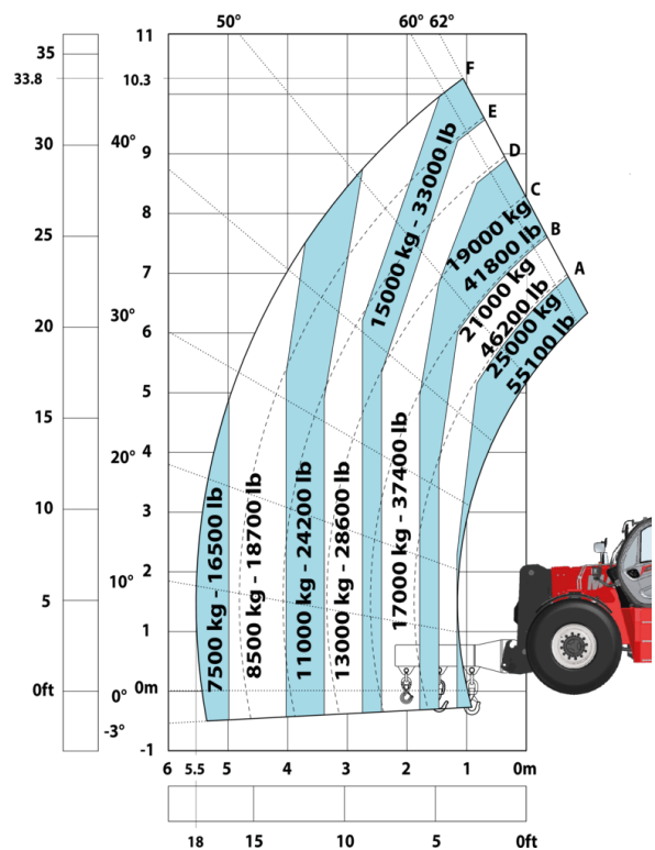
Maszyna na oponach z 3-hook wysięgnikiem 25000 kg (metryczne)
