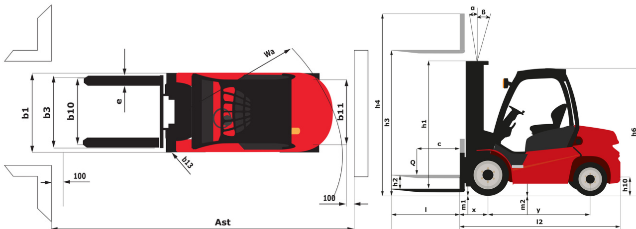
MI-X 15 G - габаритный чертеж
