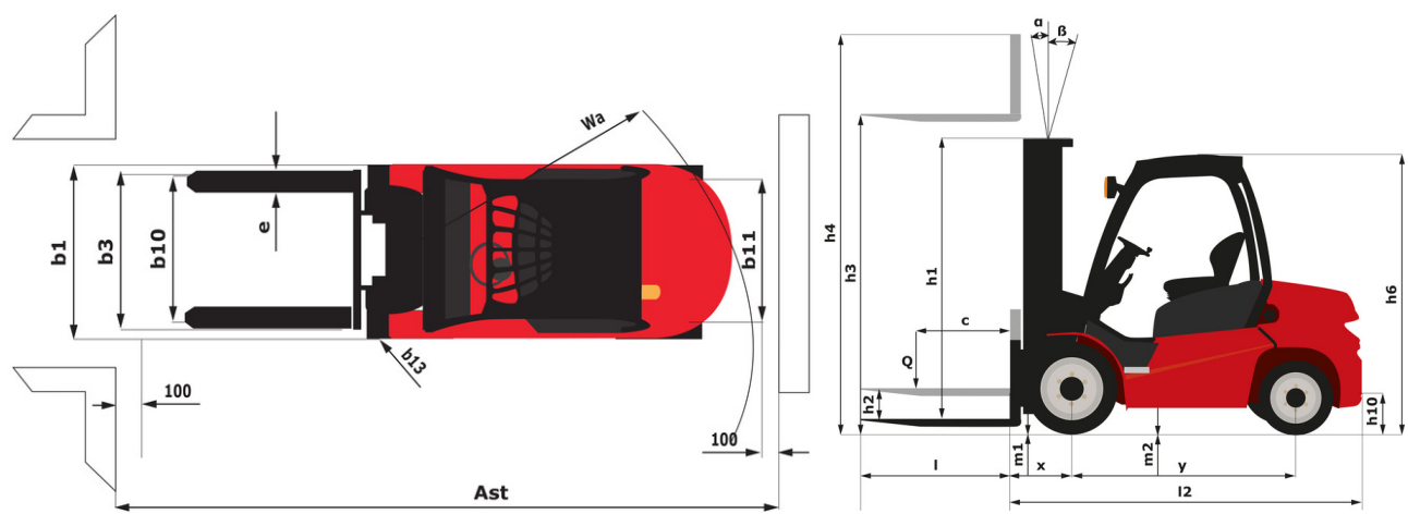
MI-X 20 G - габаритный чертеж
