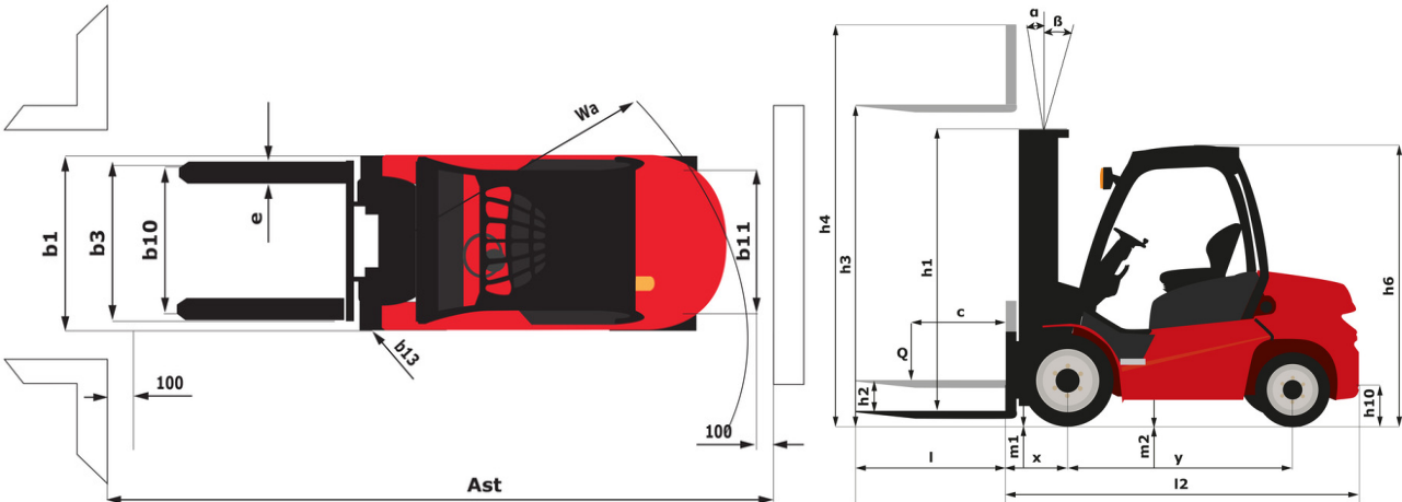
MI-X 25 D - Esquemas dimensionais
