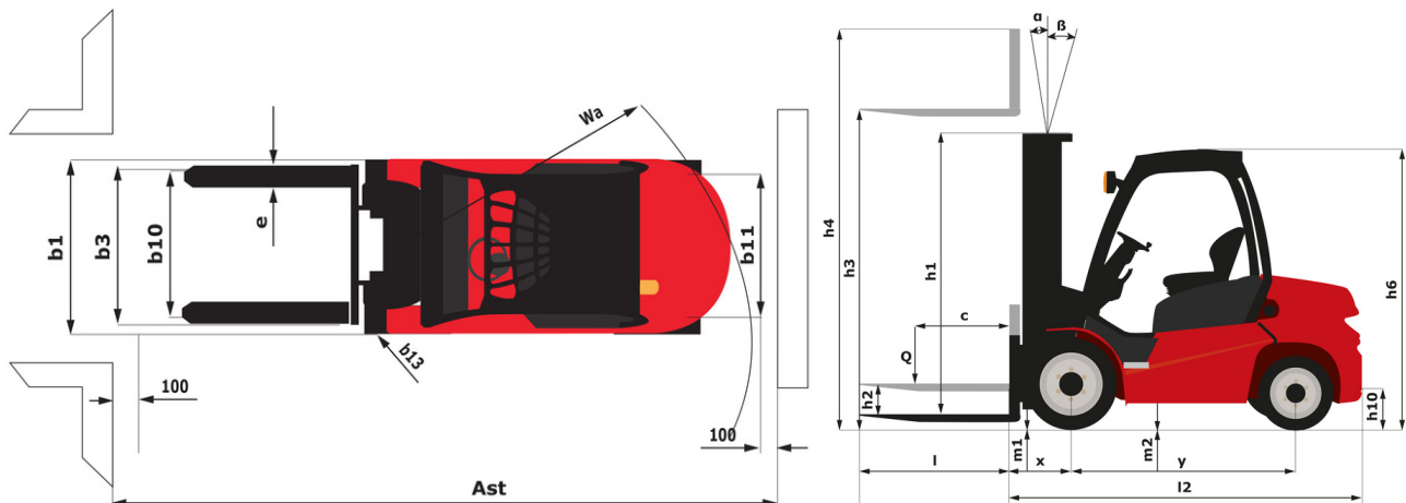
MI-X 30 D - габаритный чертеж
