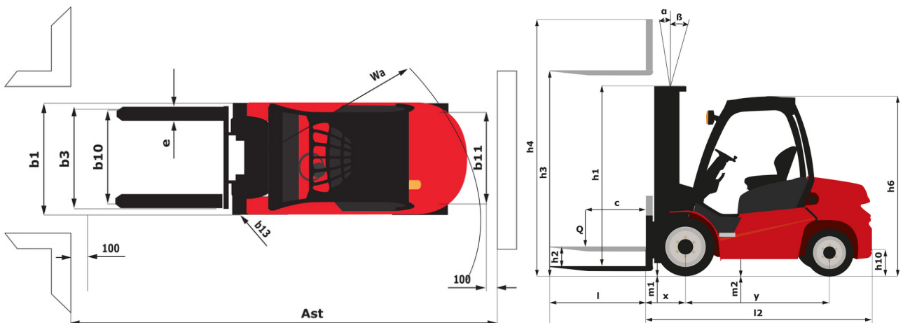
MI-X 30 G - габаритный чертеж
