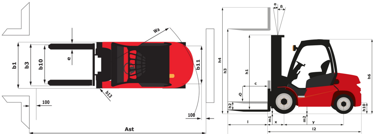
MI-X 30 G - габаритный чертеж
