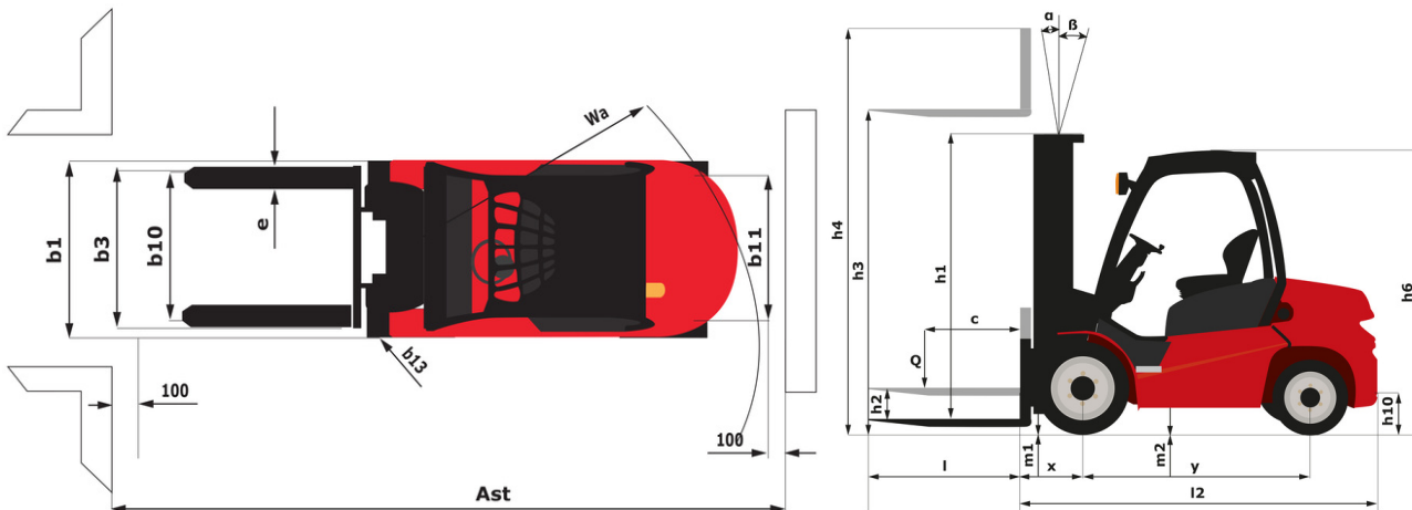
MI-X 35 D - габаритный чертёж
