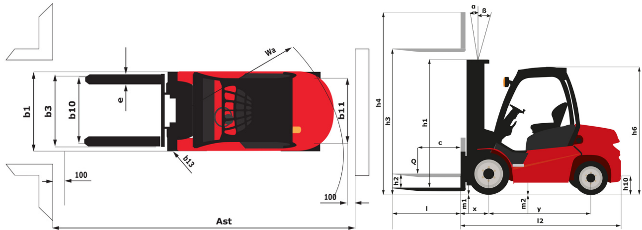
MI 45 D ST5 - Maßzeichnung
