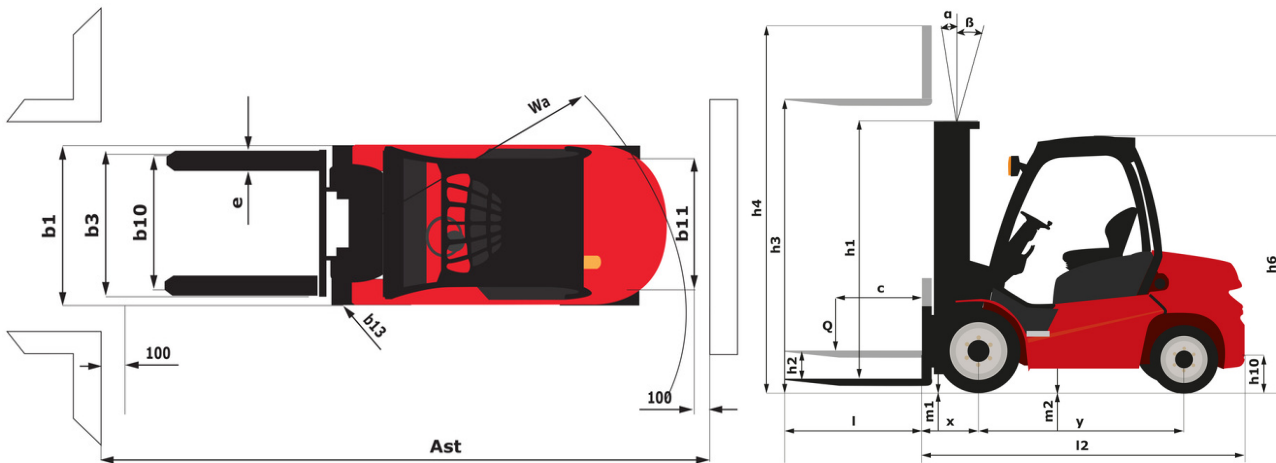
MI 50 LD ST5 - Rysunek wymiarowy
