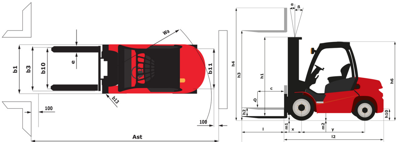
MI 70 D ST5 - Diagrama dimensional
