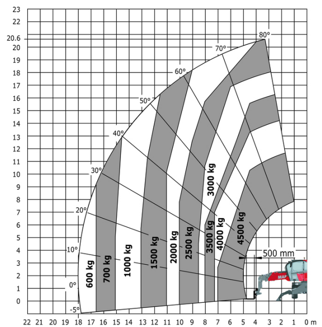
Drehung auf abgesenkten Stützen mit Gabeln
