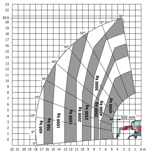
Drehung auf abgesenkten Stützen mit Gabeln
