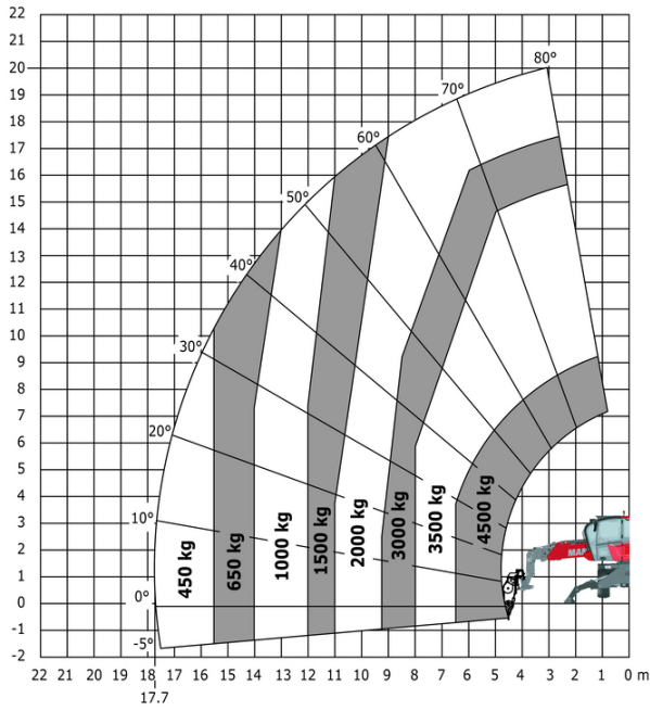
Drehung auf abgesenkten Stützen mit Winde 5000 kg
