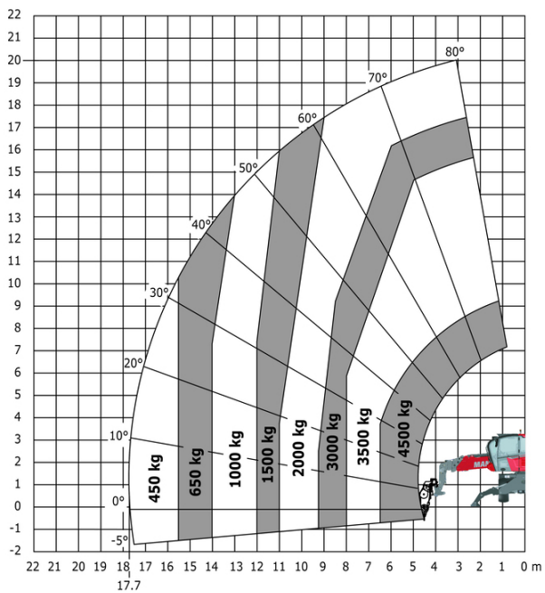
Drehung auf abgeseenkten Stützen mit Winde 5000 kg
