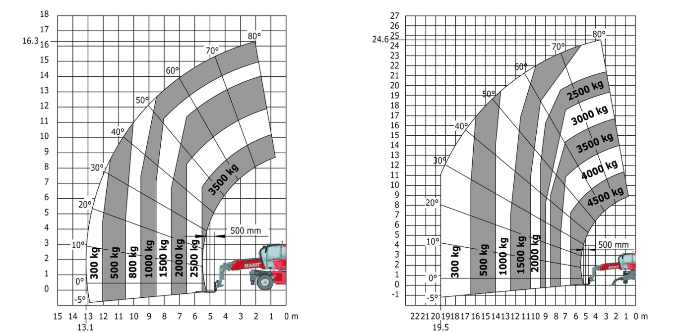
Máquina sobre neumáticos con horquillas
