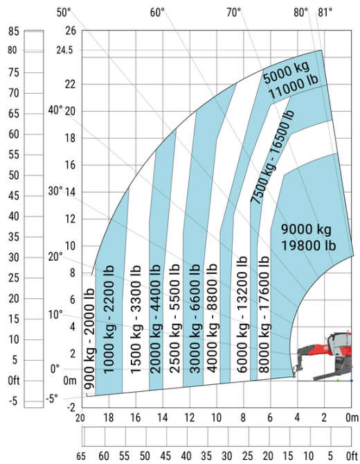
Máquina sobre estabilizadores rebaixados com gancho 9000 kg (Metric)
