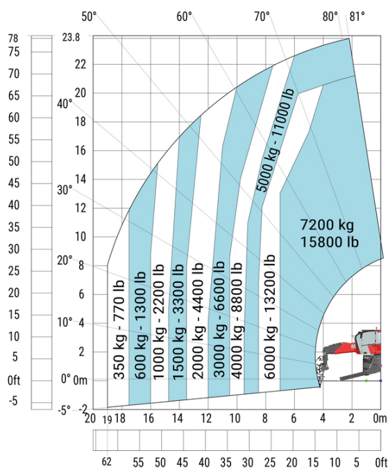
Máquina sobre estabilizadores rebaixados com guincho de 7200 kg (métrico)
