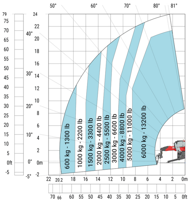
Máquina sobre estabilizadores rebaixados com guincho 6000 kg (Metric)
