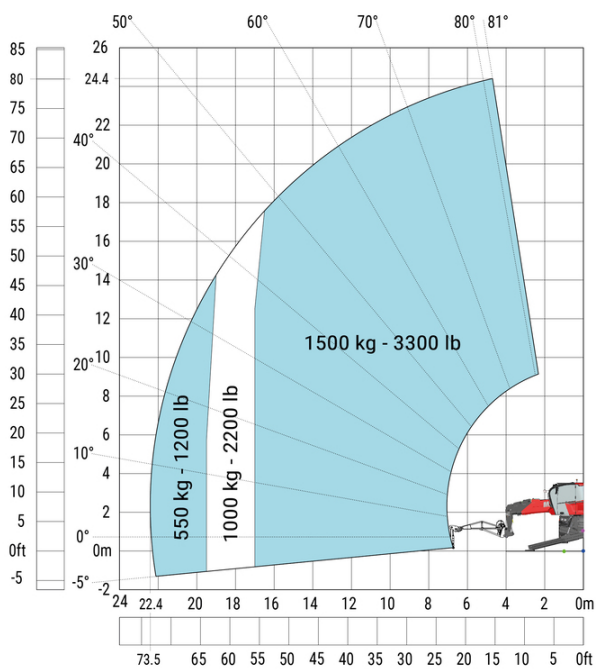
Máquina sobre estabilizadores rebaixados com lança de 1500 kg Métrico
