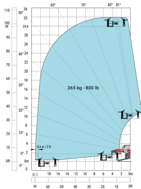
Machine sur stabilisateurs abaissés avec nacelle 365 kg (Métrique)
