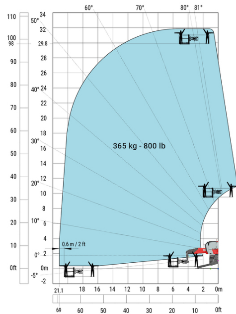
Máquina sobre estabilizadores rebaixados com plataforma de 365 kg Métrico
