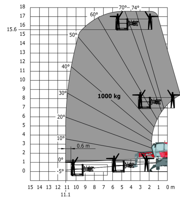
Machine sur stabilisateurs abaissés avec nacelle 1000 kg
