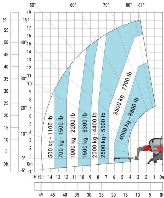
Máquina com estabilizadores acionados com jib (Métrico)
