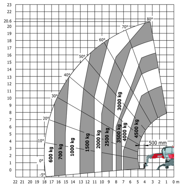
Máquina em estabilizadores abaixados com garfos métricos
