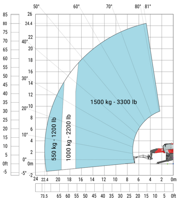
Máquina sobre estabilizadores rebaixados com lança métrica de 1500 kg
