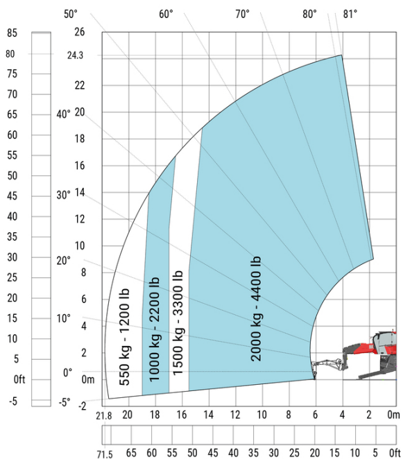
Rotação sobre estabilizadores com extensão (Potence) de 2000 kg (Métrico)
