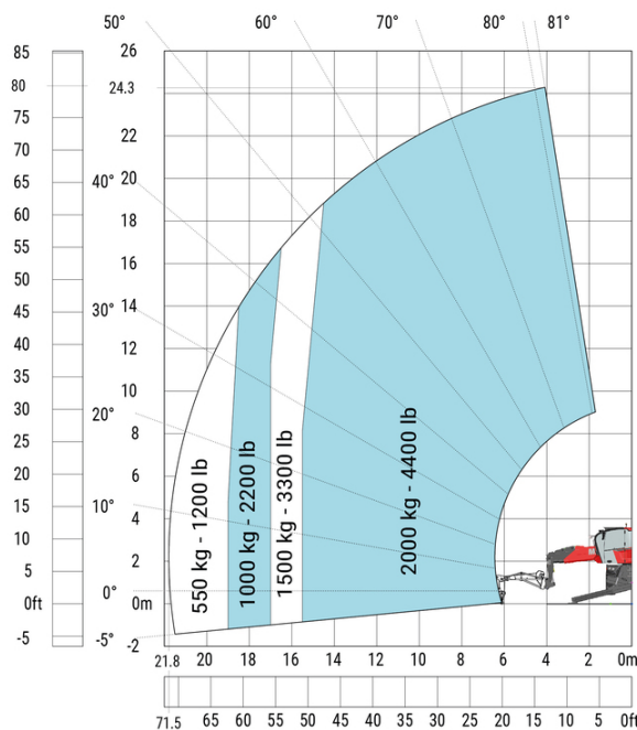
Машина при опущенных аутригерах со стрелой 1500 кг Машина на установленных аутригерах с весом на стреле 2000 кг, метрическая система мер
