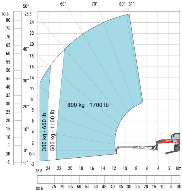
Машина на опущенных аутригерах с выдвжной кран-балкой с лебедкой, метрическая система мер
