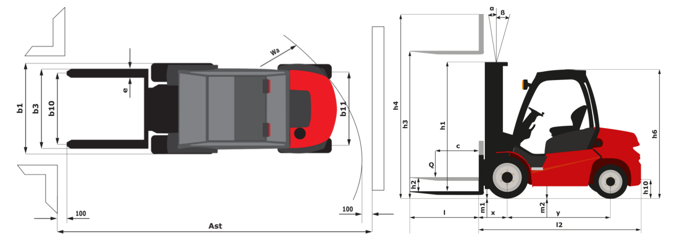
MSI-X 35 - габаритный чертеж
