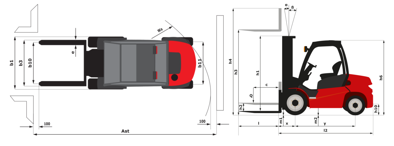
MSI-X 35 - габаритный чертёж
