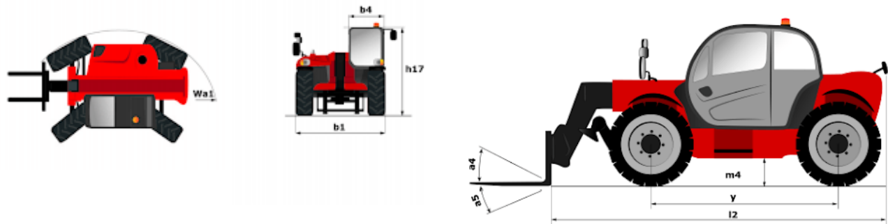
MTA 12055 serie 3 - Dimensional drawing
