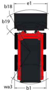
2100V - 寸法図
