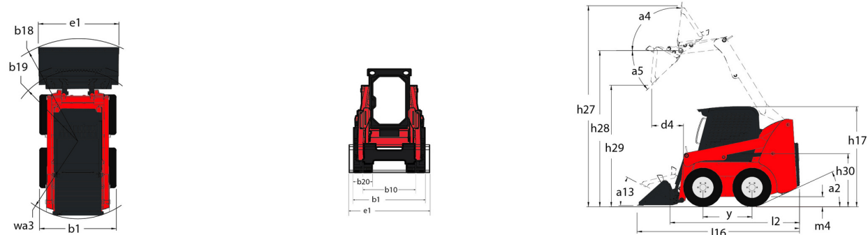
1650R - габаритный чертеж
