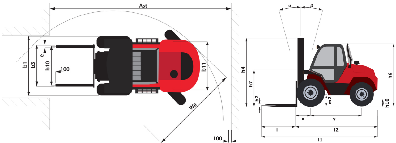
М-Х 50-4 - габаритный чертеж
