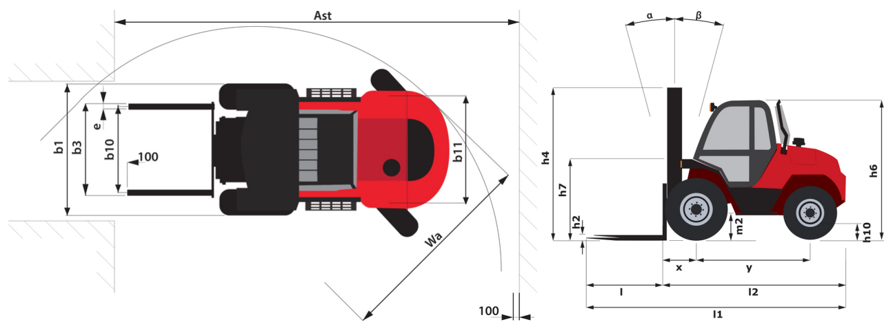
М-X 70-2 - габаритный чертеж
