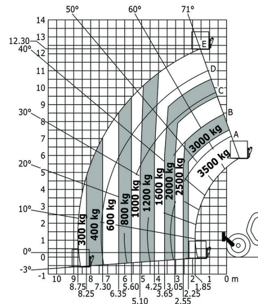
Machine op banden met vorken - met nivellering
