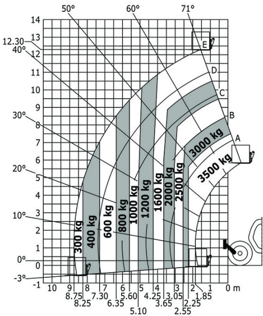
Máquina sobre pneus com garfos - com nivelamento (métrico)
