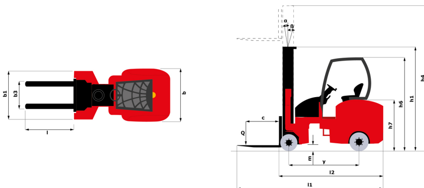
EMA II 18 HL-2 - габаритный чертеж
