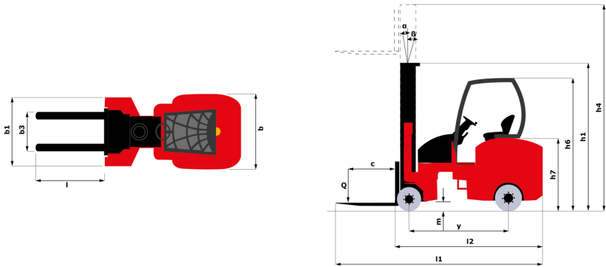
EMA II 13 - Rysunek wymiarowy
