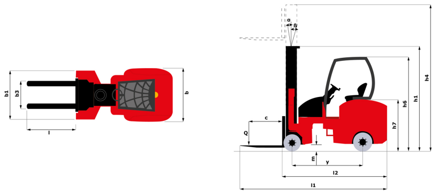
ЕМА II 20 - габаритный чертеж
