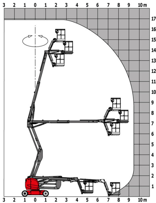
Wykres udźwigów
