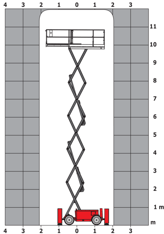
Gráfico da carga para plataforma elevatória (métrico)
