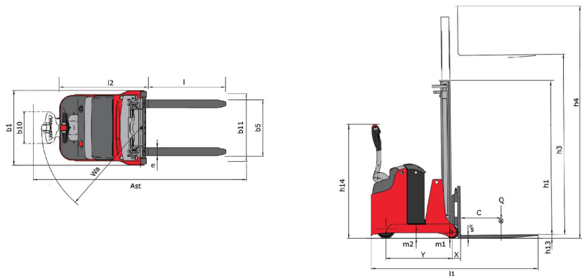
ES-C 504 - Diagrama dimensional
