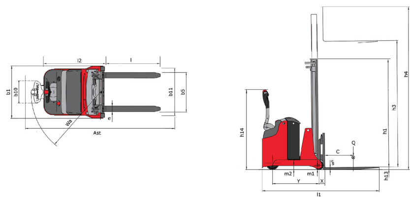
ES-C 507 - габаритный чертеж
