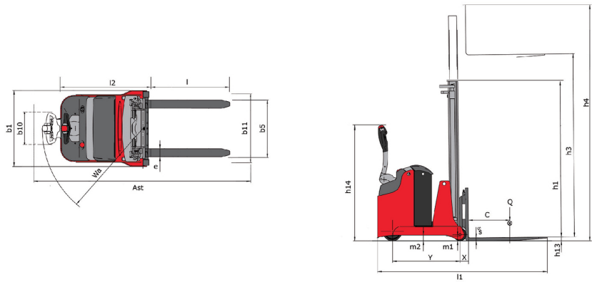
ES-C 510 - Diagrama dimensional
