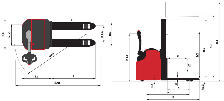
ES 616 LI - Dimensional drawing
