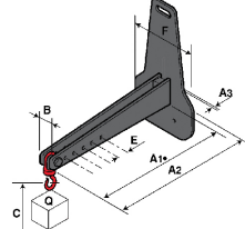
POT 500
