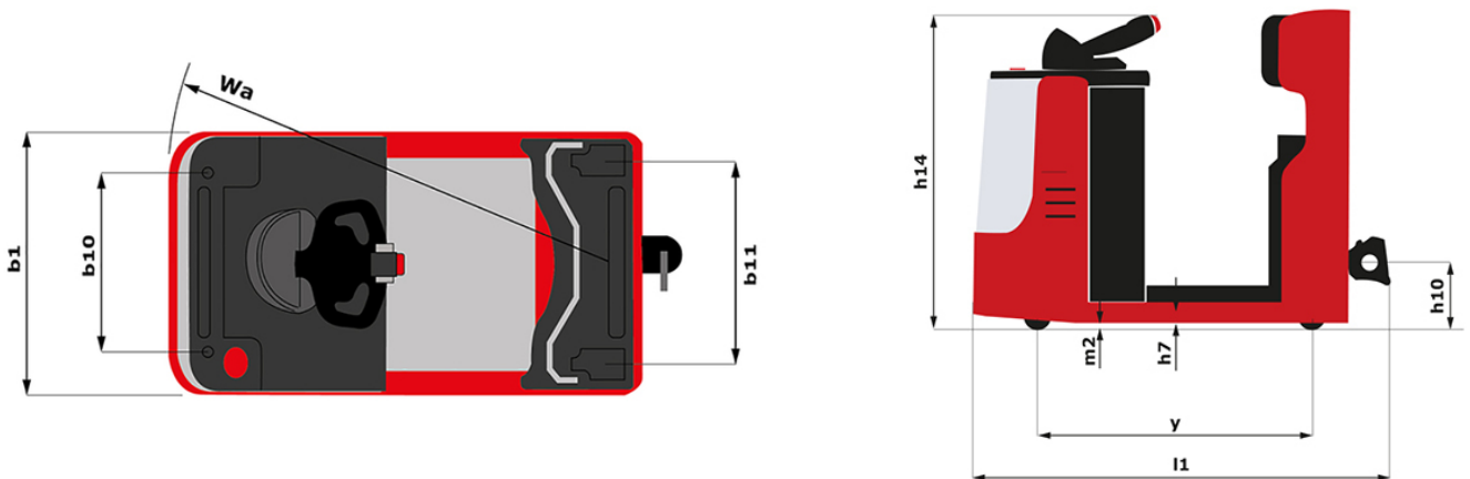
CT 50 - 寸法図
